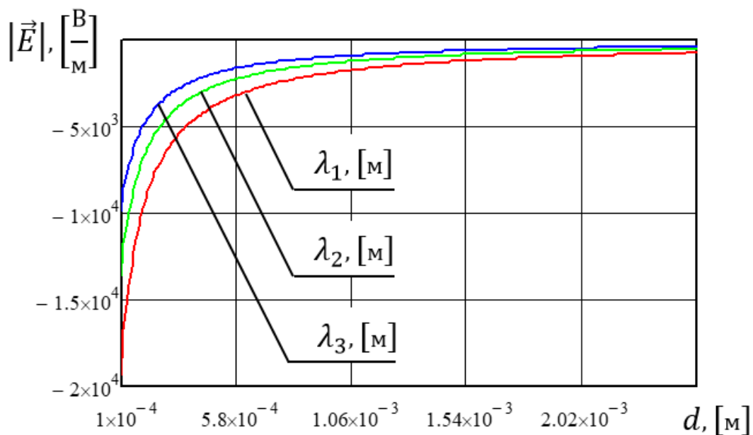
Рисунок 3 – График зависимости вида |\vec{E}| = f(d)
