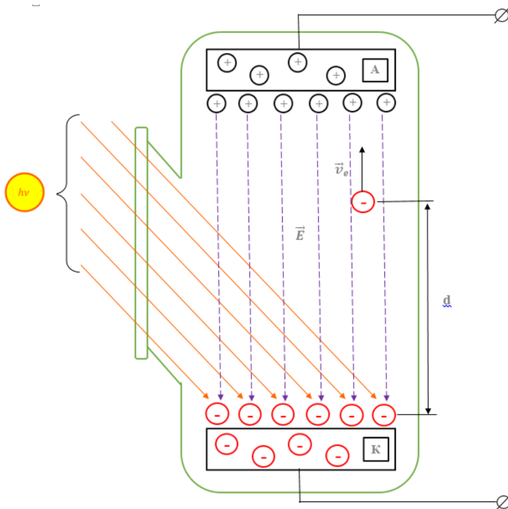
Рисунок 2 – Схема эксперимента по исследованию внешнего фотоэффекта
